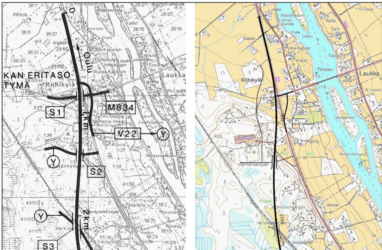
Kuva 28. Ohikulkuvaihtoehdon ve 1 liittymäratkaisut Riihikylän kohdalla. Vasemmalla vanhan yleissuunnitelman ratkaisu ja oikealla uusi ratkaisu.
