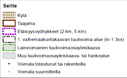
Kuva 6. Tuulivoima-alueet Kalajoen Mehtäkylän ympäristössä.
