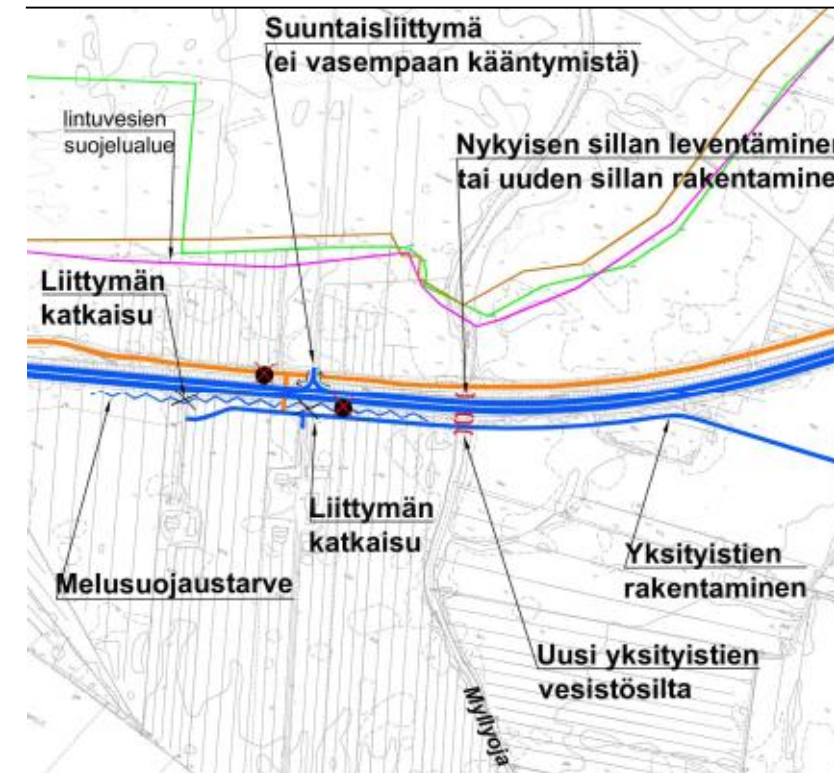
Kuva 26. Luonnos nelikaistaisesta Lentokentäntiestä ja linjaosuuden liittymävaihtoehdosta. (Karttapohja Oulun kaupunki).
