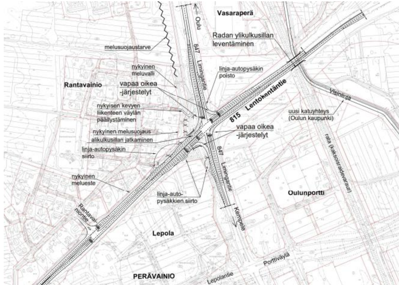
Kuva 21. Luonnos Lentokentätien ja Oulunlahdentien lisäkaistasta ja Limingantien liikennevaloliittymän vapaa-oikea -järjestelyistä. (Karttapohja Oulun kaupunki).
