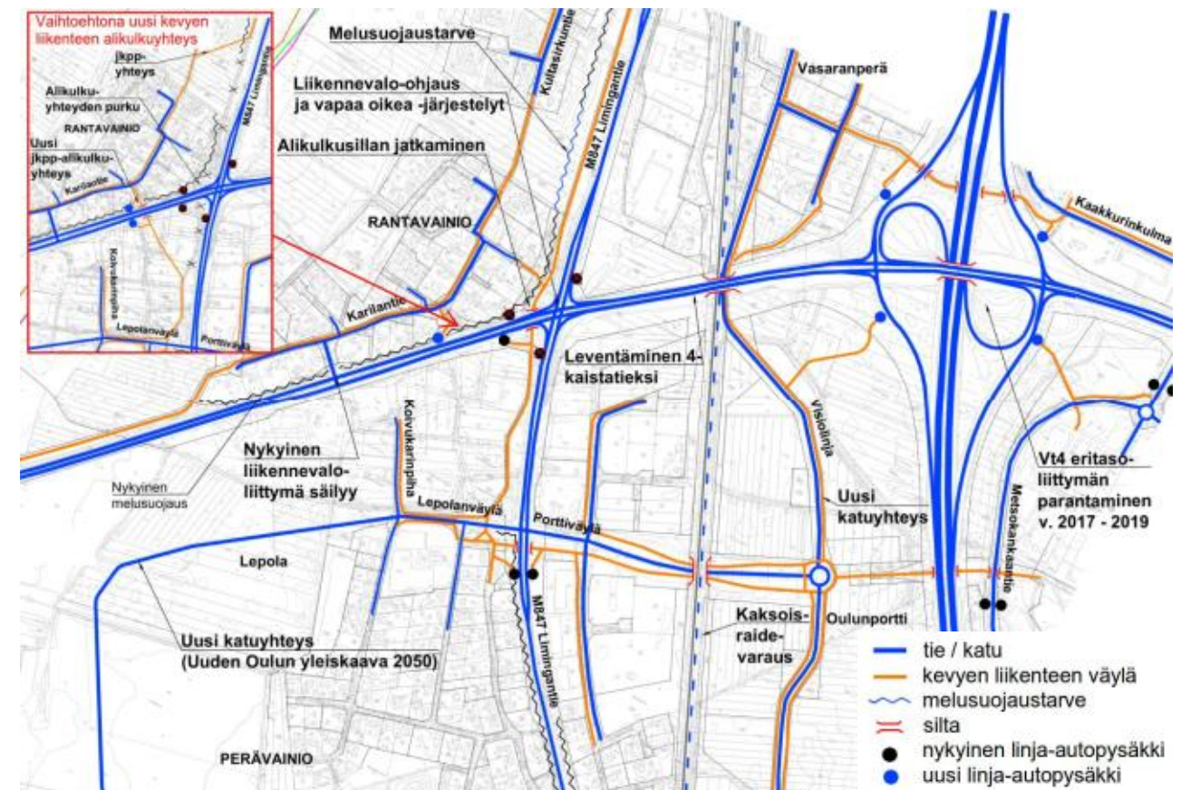
Kuva 20. Luonnos Rantavainion ja Limingantien ympäristön liikenneverkosta ja tasoliittymäratkaisusta VE 1. (Karttapohja Oulun kaupunki).
